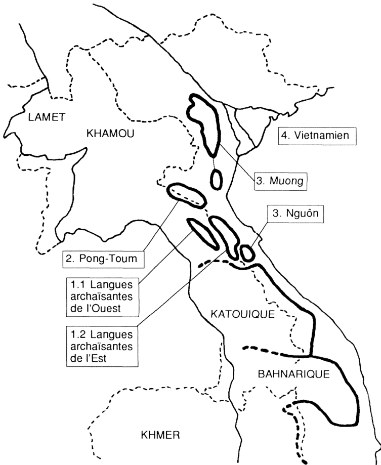
Repartition des langues viet-muong.
